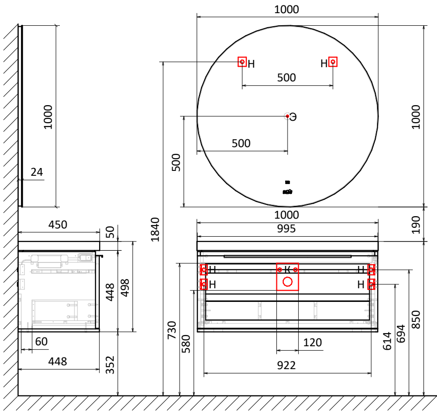
Зеркало Solo 100 Тумба подвесная Notte100
